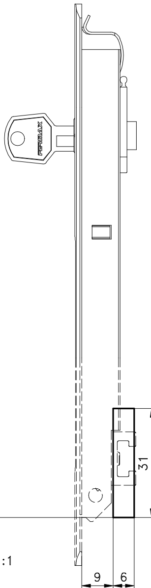
Vistas - escala 1:1
