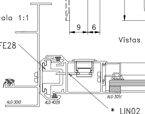
Instalação - escala 1:2
