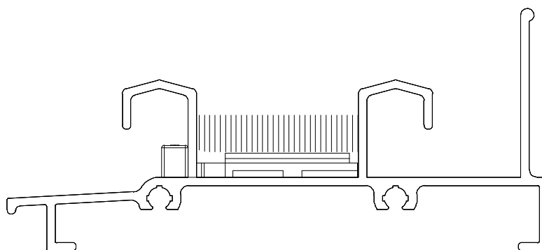
Instalação - escala 1:1
