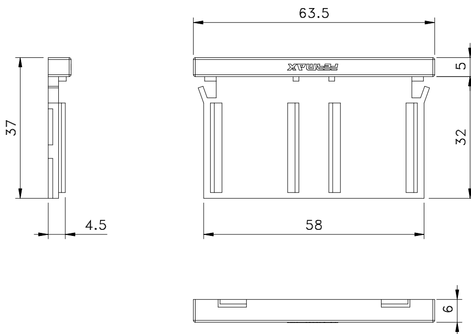
Vistas - escala 1:1
