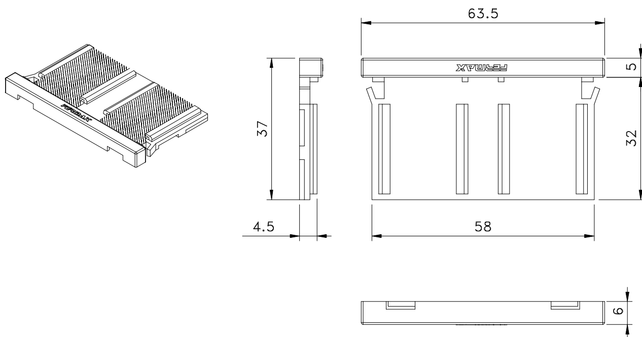
Vistas — escala 1:1
