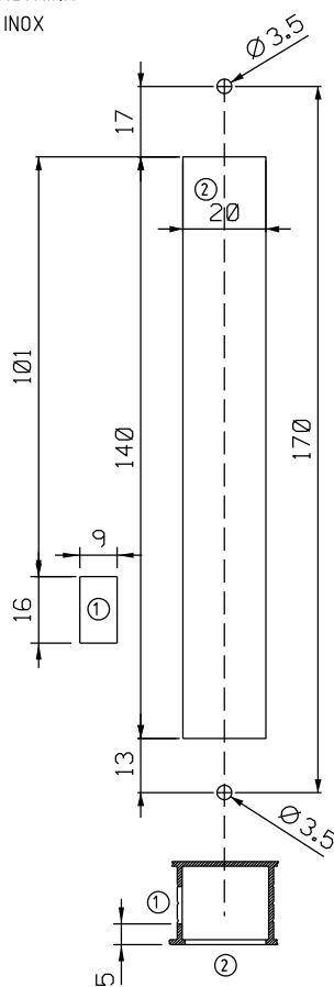
Usinagem - escala 1:2
