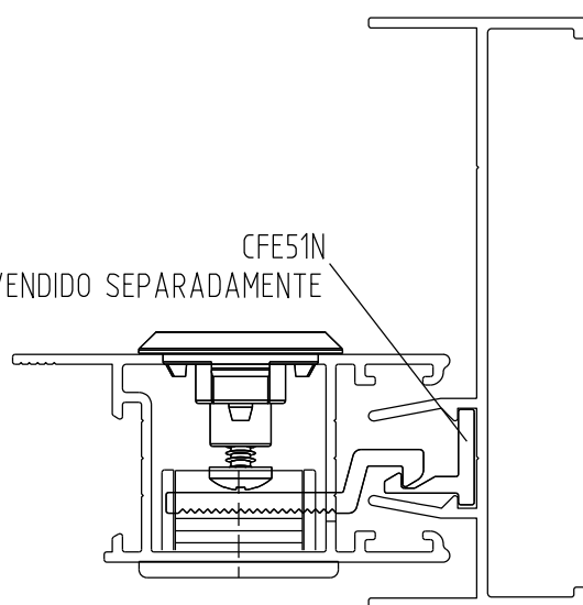
Instalação - escala 1:1
