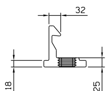
Vistas - escala 1:1
