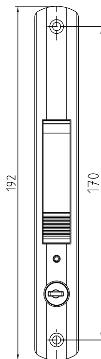
VISTAS ESCALA 1:2
