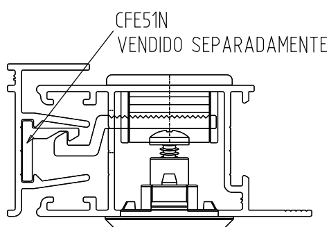
Instala231227o - escala 1:1
