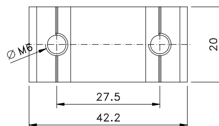
■ Vistas – escala 1:1
