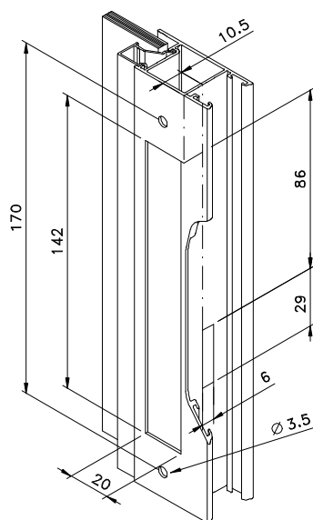
Usinagem para instalação Sem escala
