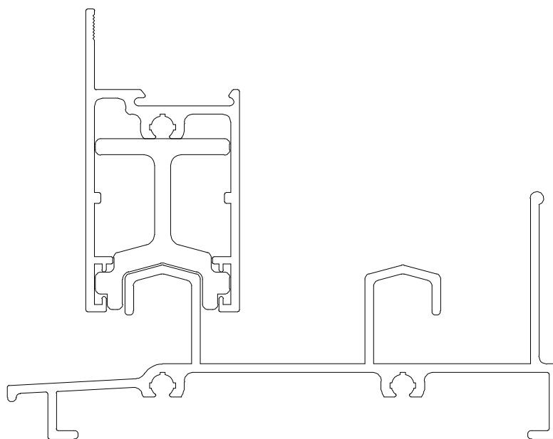
Vistas - escala 1:1
