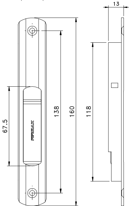
Vistas - escala 1:2
