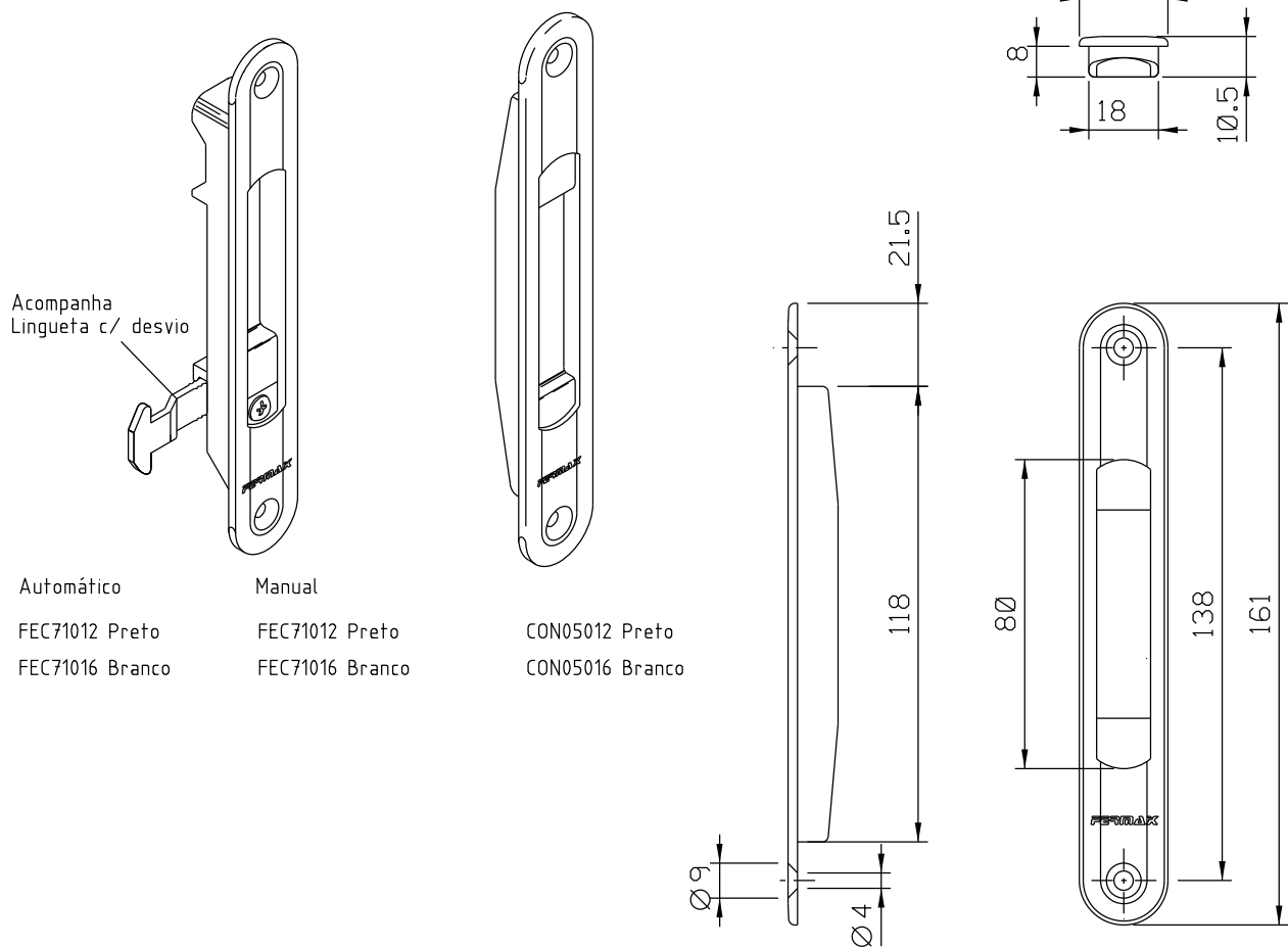
Vistas - escala 1:2
