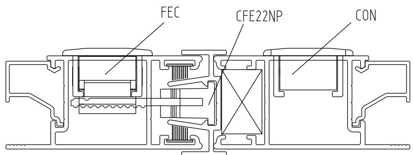
Instalação - escala 1:1
