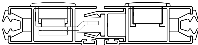
Instalação - escala 1:1
