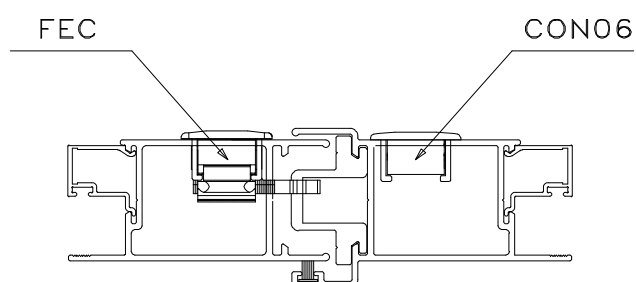
Instalação - escala 1:1
