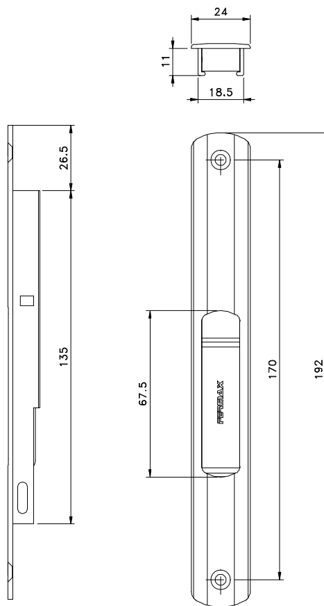
Vistas - escala 1:2
