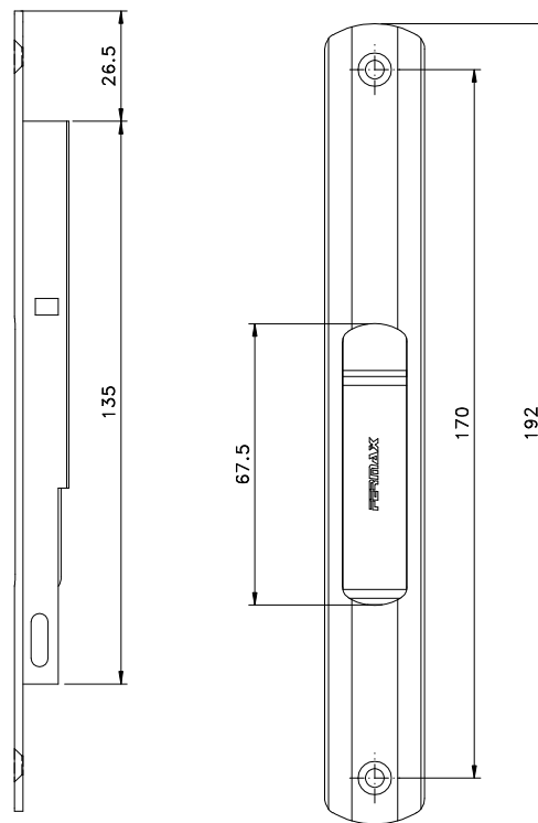
Vista – escala 1:2
