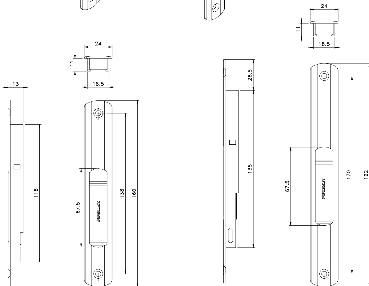
Vistas - escala 1:2
