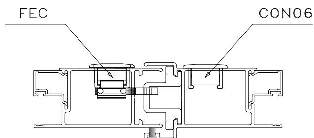
Instalação - escala 1:1
