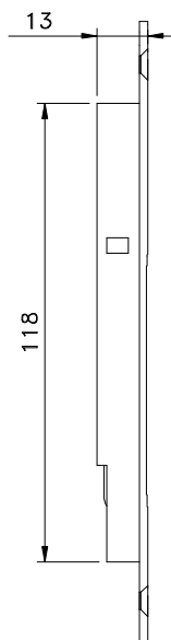
Vistas - escala 1:2
