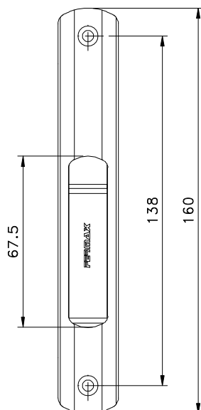
Vistas - escala 1:2
