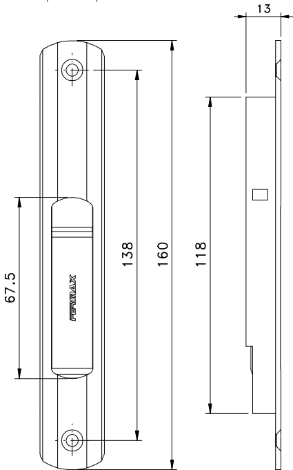
Vistas - escala 1:2
