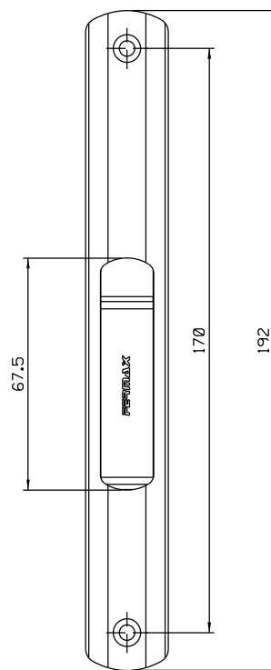
Vistas - escala 1:2
