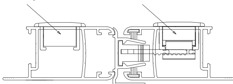
Instalação - escala 1:1
