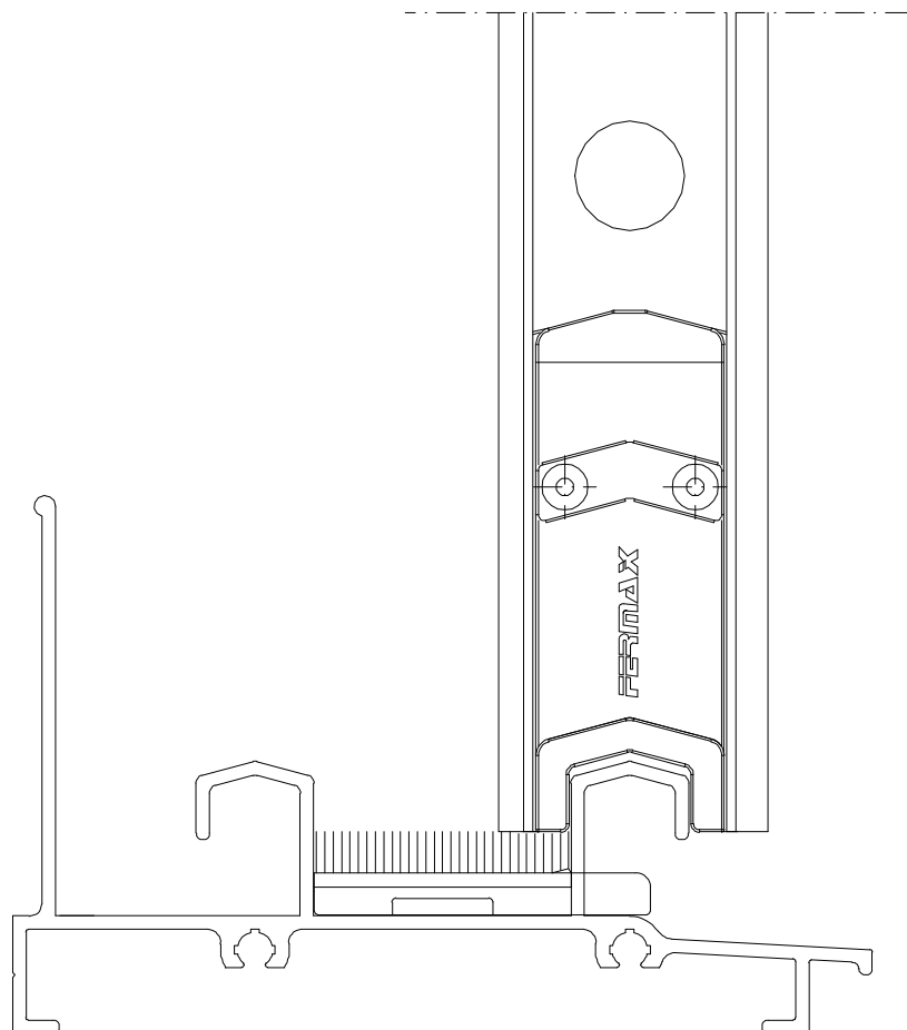
Instalação - escala 1:1
