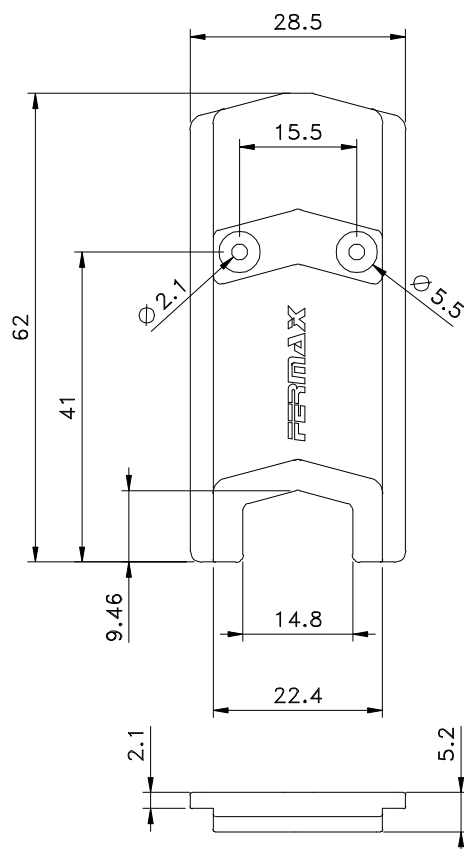
Vistas - escala 1:1
