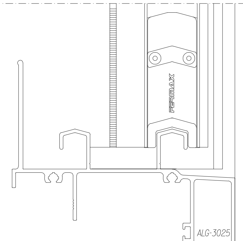
Instalação - escala 1:1
