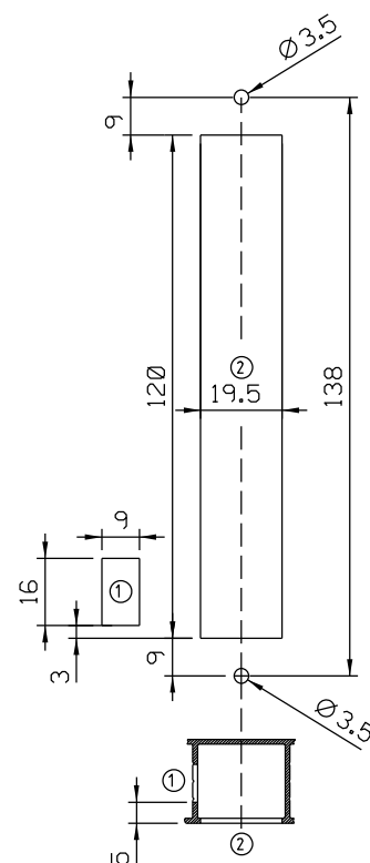
Usinagem - escala 1:2
