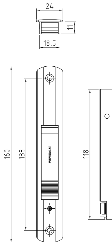
VISTAS ESCALA 1:2
