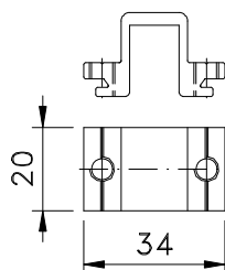
Vistas - sem escala
