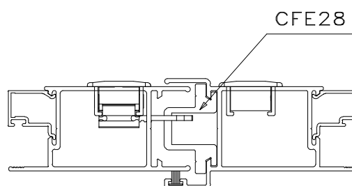
Instalação - escala 1:2
