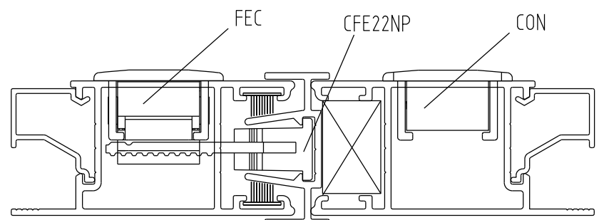
Instalação - escala 1:1
