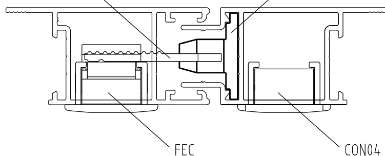
Instalação - escala 1:1
