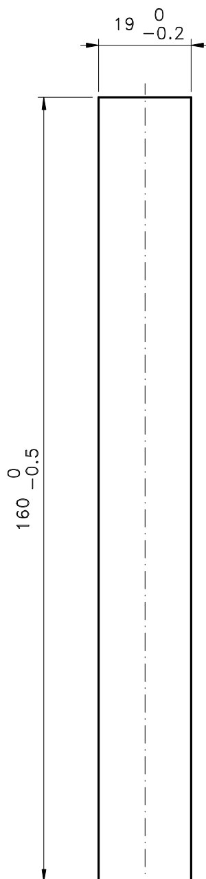
Usinagem - escala 1:1
