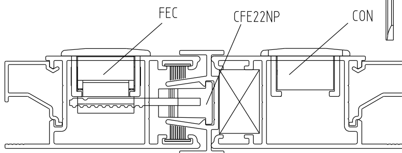
Usinagem - escala 1:1
