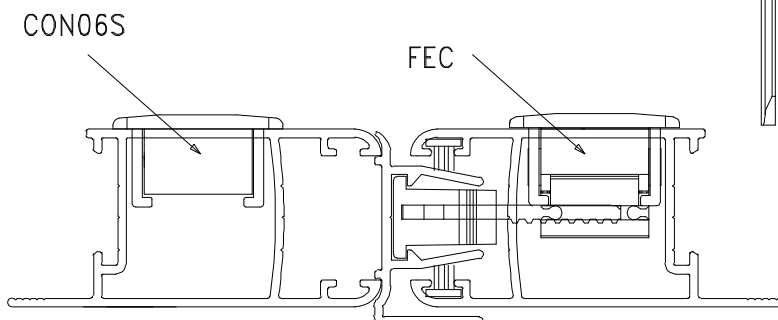
Instalação - escala 1:1
