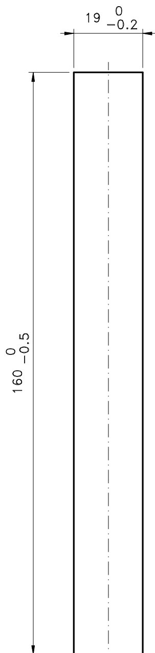
Usinagem - escala 1:1
