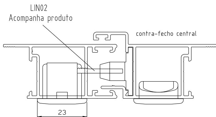
Instalação - escala 1:1
