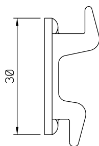
Contra-fecho central Escala 1:1
