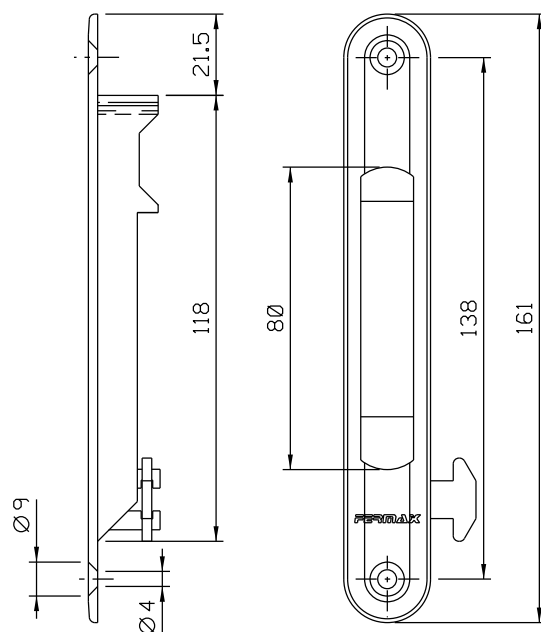
Vistas - escala 1:2
