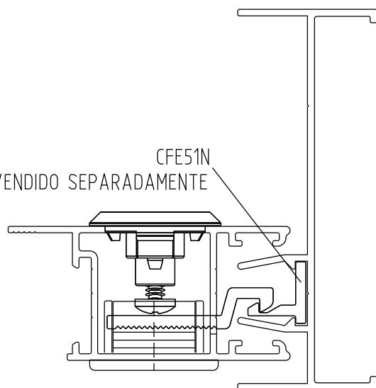
Instalação - escala 1:1
