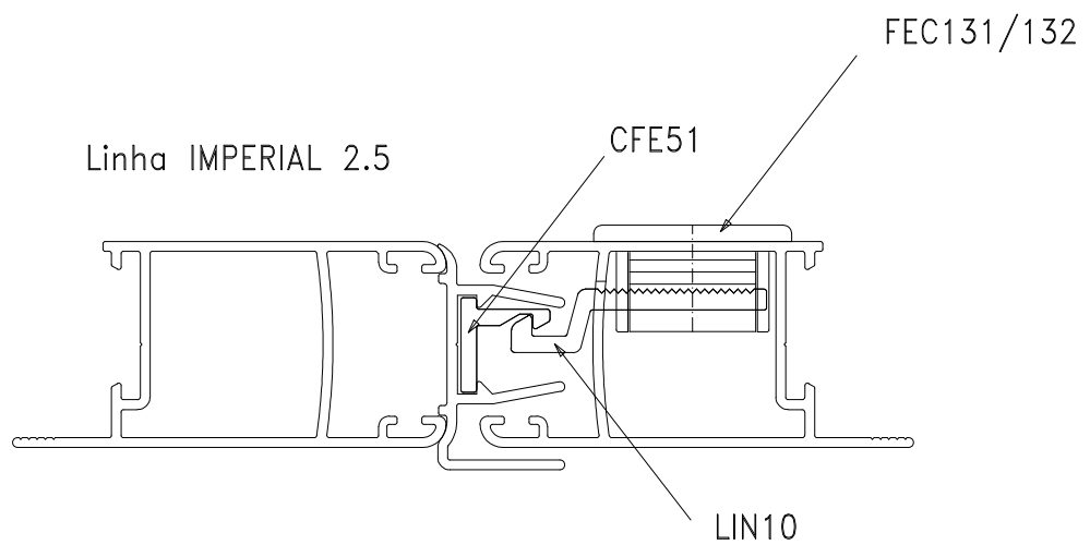
Instalação - escala 1:1
