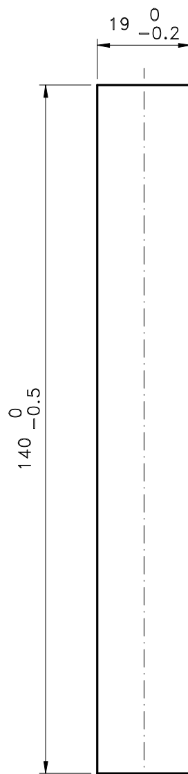
Usinagem - escala 1:1
