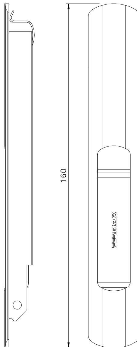
Vistas - escala 1:1
