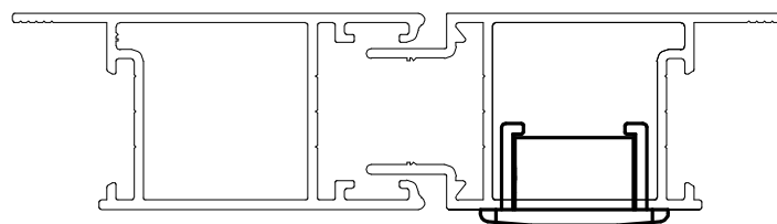
Instalação - escala 1:1
