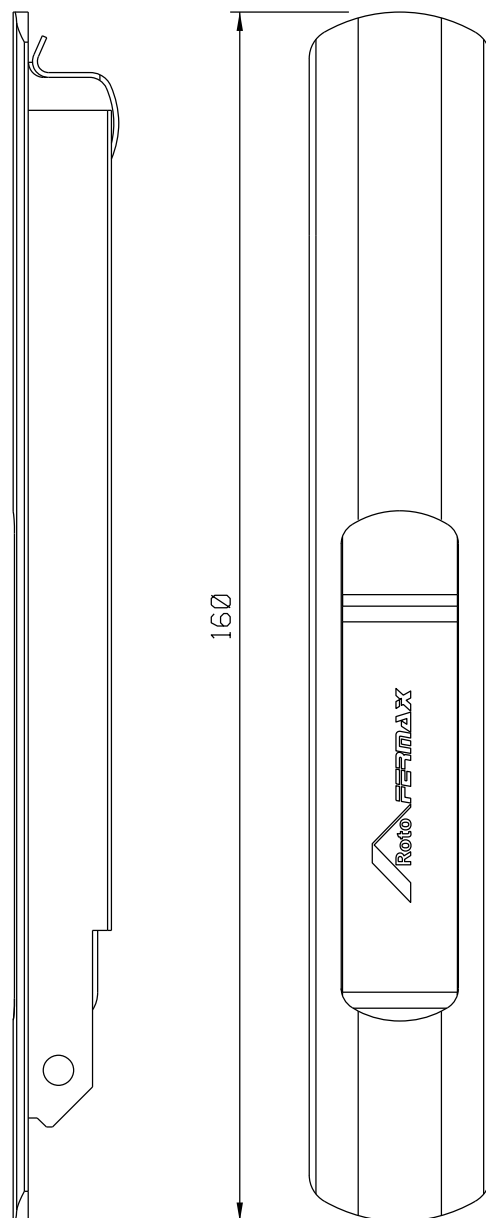
Vistas - escala 1:1
