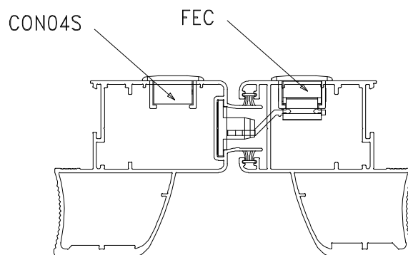
Instalação - escala 1:2
