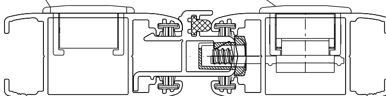
Instala**o - escala 1:1
