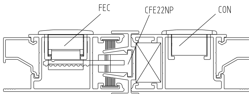
Vistas - escala 1:1
