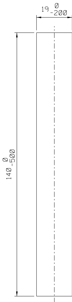
Usinagem - escala 1:1
