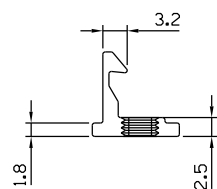
Vistas - escala 1:1
