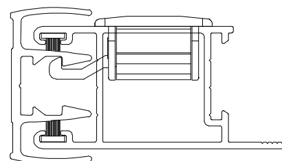
Vistas – escala 1:1
