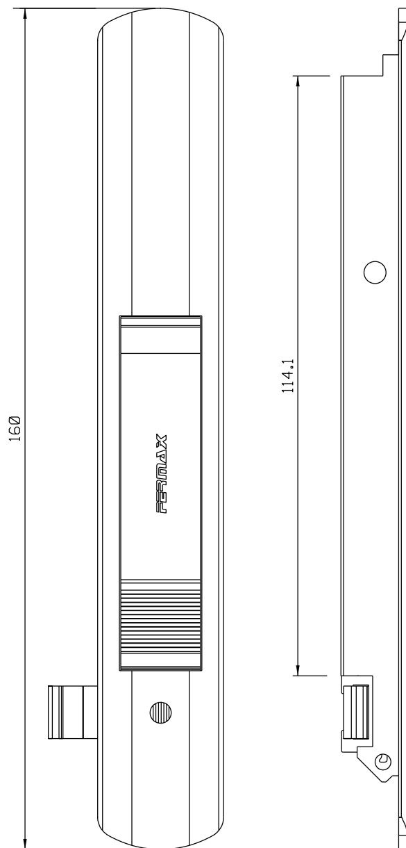
Vistas - escala 1:1
