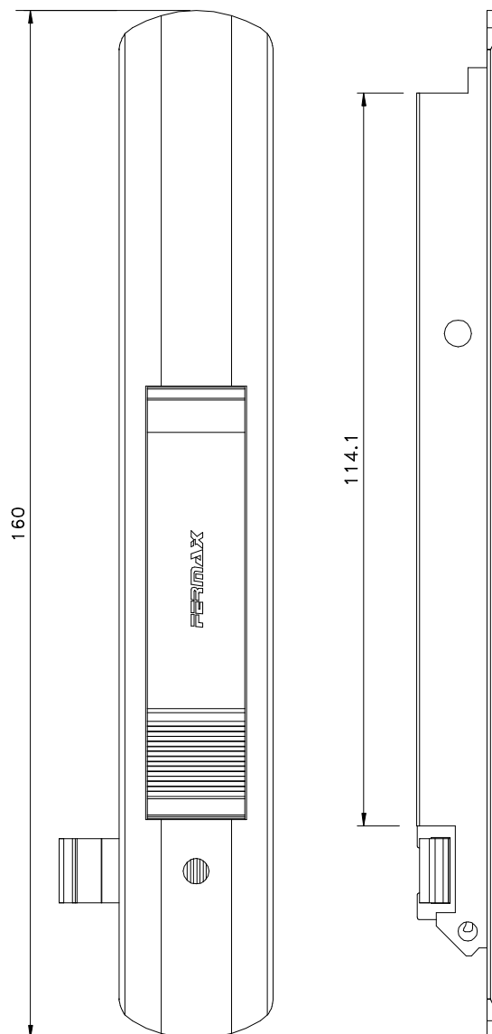
Vistas - escala 1:1
