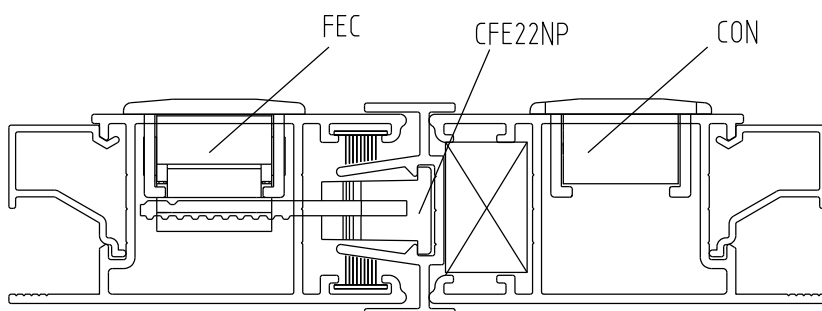
Instalação - escala 1:1
