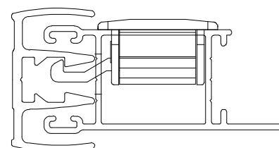
Vistas - escala 1:1
