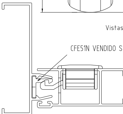
Instalação - escala 1:1
