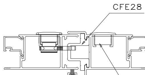
Usinagem para instalação Sem escala
