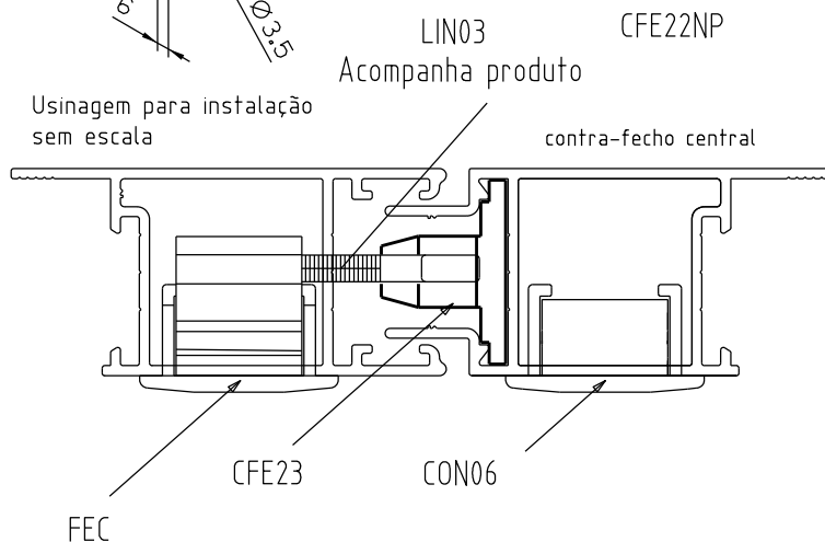
Instalação - escala 1:1
