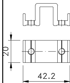
Vistas - sem escala
