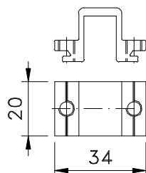
Vistas - sem escala
