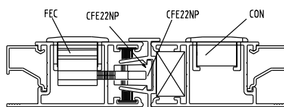
Instalação - escala 1:2
