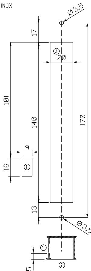
Usinagem - escala 1:2
