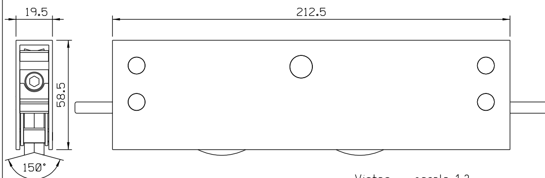
Vistas - escala 1:2
