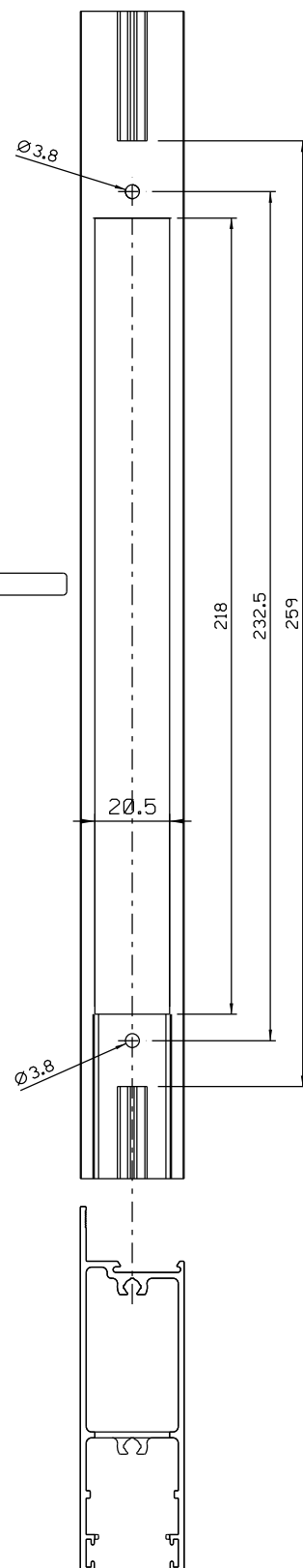
Usinagem - escala 1:2
