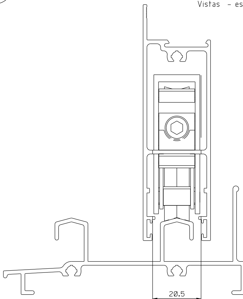
Instalação - escala 1:1
