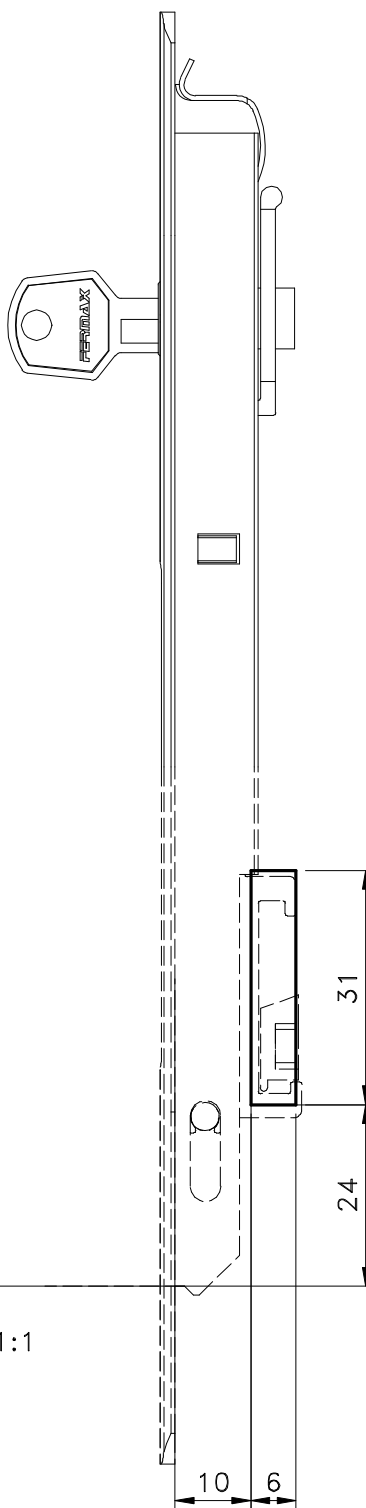
Vistas - escala 1:1
