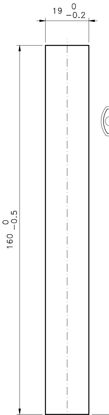
Usinagem - escala 1:1
