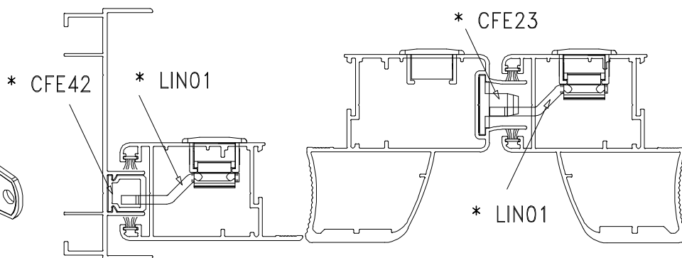
Instalação - escala 1:2
