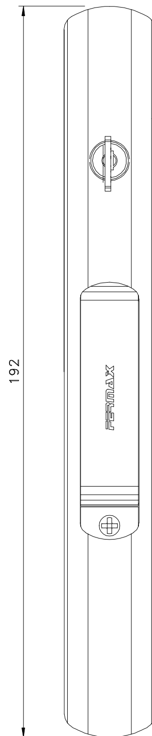
Vistas - escala 1:1
