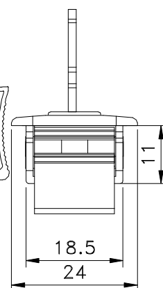
Instalação - escala 1:2
