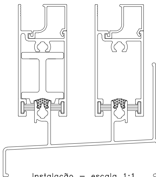
Instalação – escala 1:1
