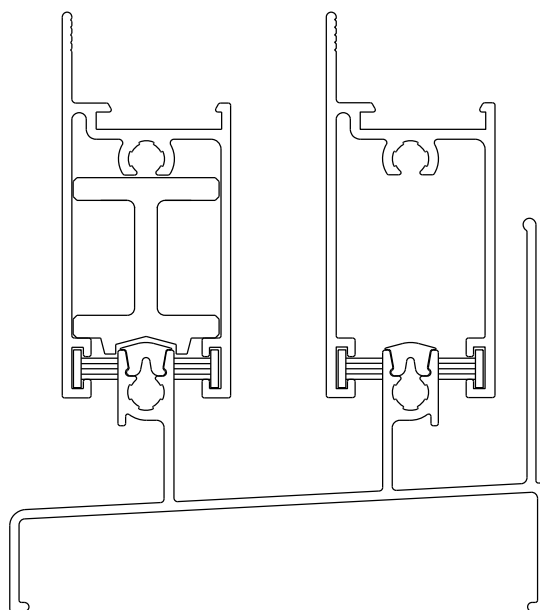
Instalação - escala 1:1
