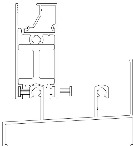
Instalação – escala 1:1
