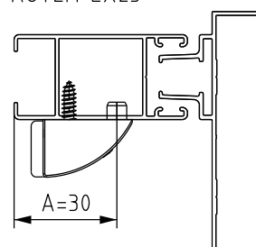
INSTALAÇÃO ESCALA 1:2
