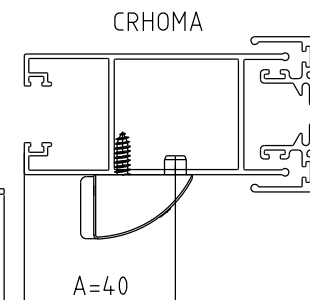
INSTALAÇÃO ESCALA 1:2
