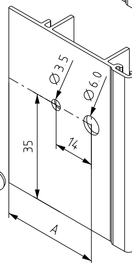
DETALHE DE USINAGEM SEM ESCALA
