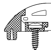
INSTRUÇÃO PARA COLOCAÇÃO DO BATEDOR
