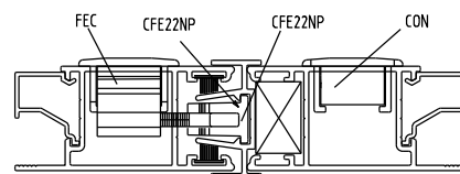
Instalação - escala 1:2
