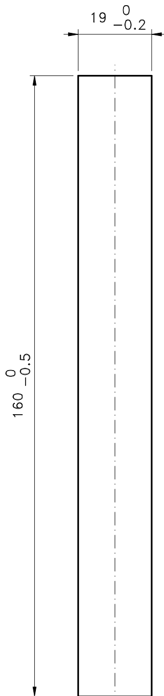
Usinagem - escala 1:1
