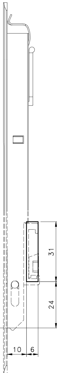
* CFE22 Vistas - escala 1:1
