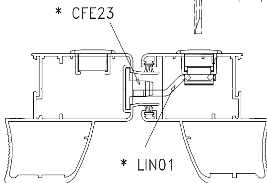
Usinagem - escala 1:1
