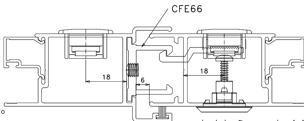
Instalação escala 1:1
