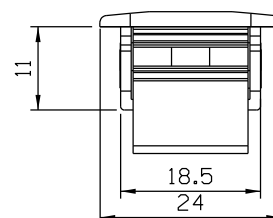
Instalação - escala 1:2
