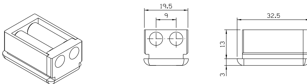
Vistas - escala 1:1
