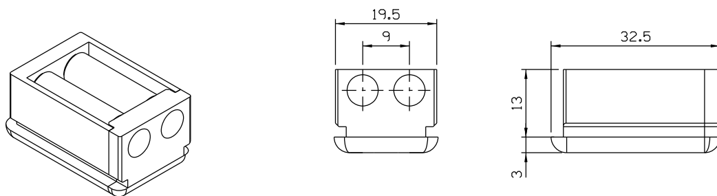
Vistas - escala 1:1
