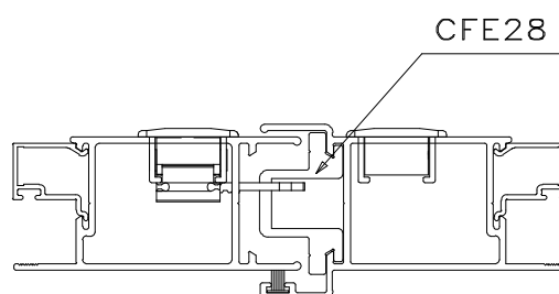
Instalação - escala 1:2
