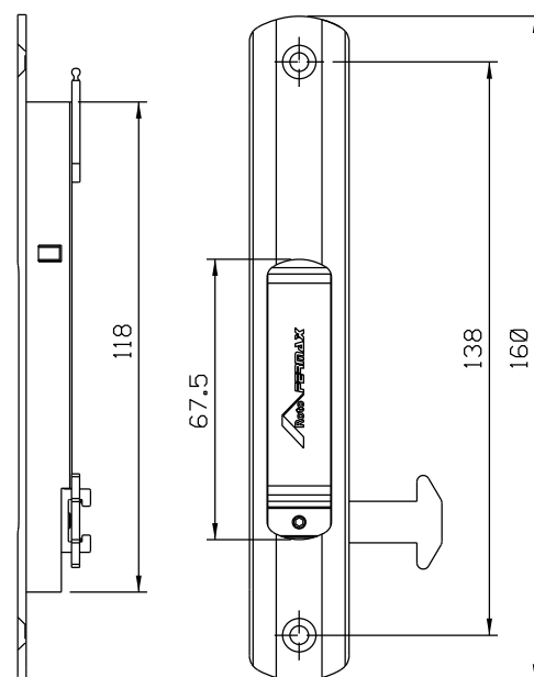
Vistas - escala 1:2
