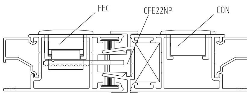
Instalação - escala 1:1
