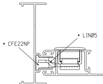
Instalação - escala 1:1
