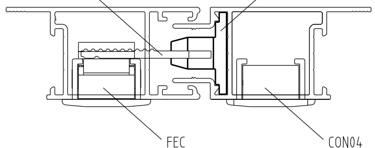
Instalação - escala 1:1
