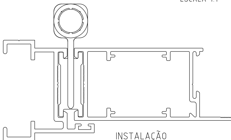
VISTAS ESCALA 1:1
