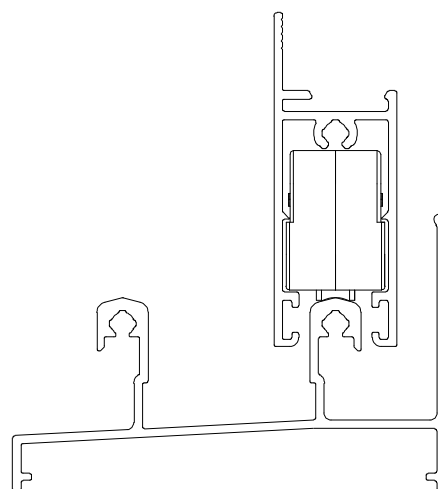
Instalação — escala 1:1
