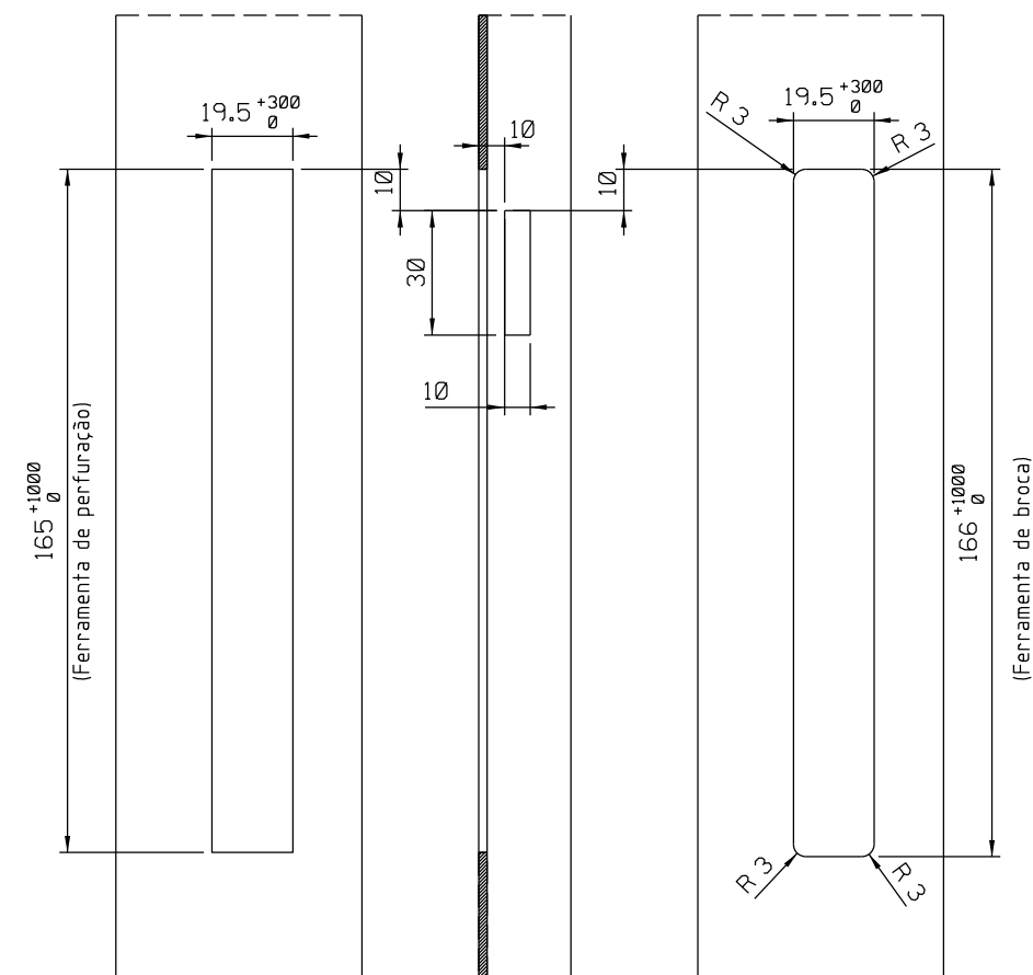
Usinagem – escala 1:2
