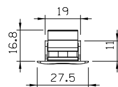
Vista - escala 1:2
