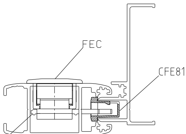
Instalação - escala 1:1
