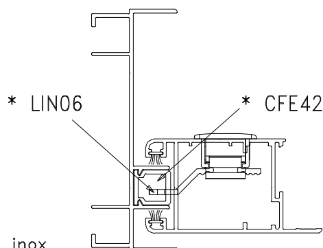
Usinagem — escala 1:1
