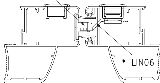
Instalação — escala 1:2
