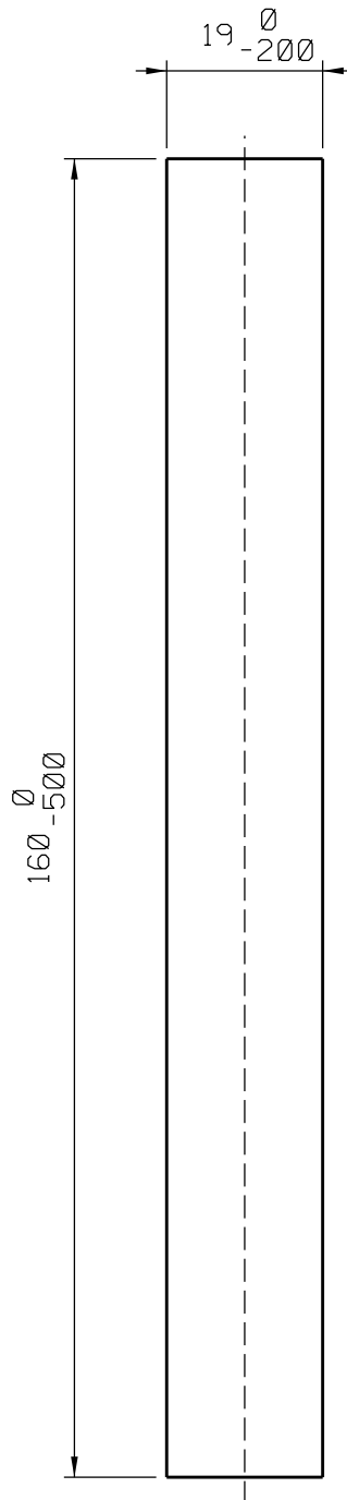
Usinagem - escala 1:1
