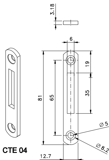
Vista - escala 1:2
