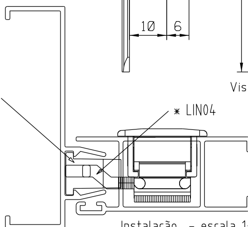
Instalação - escala 1:1
