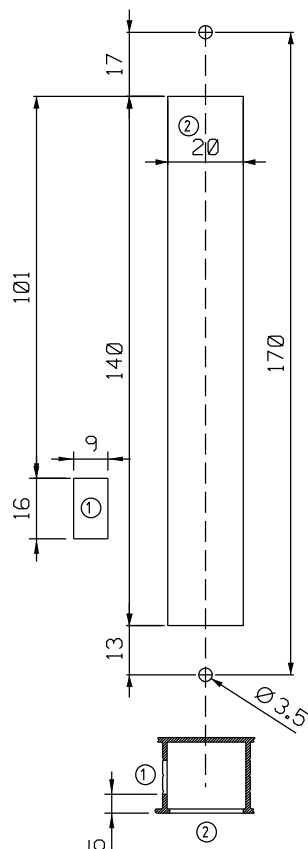
USINAGEM - ESCALA 1:2
