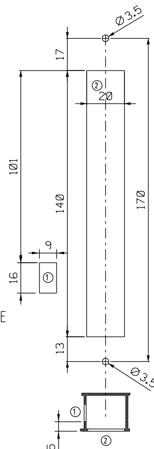
Usinagem - escala 1:2
