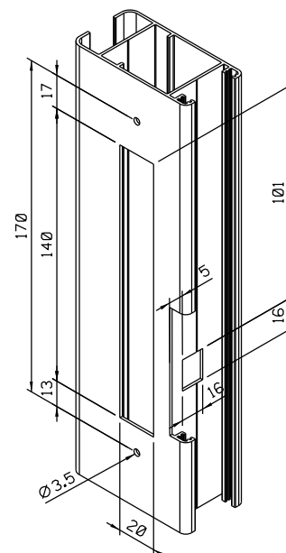
USINAGEM Sem escala
