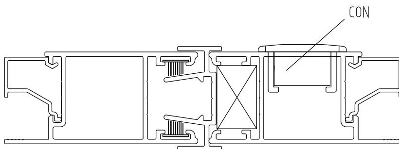
Instalação - escala 1:1
