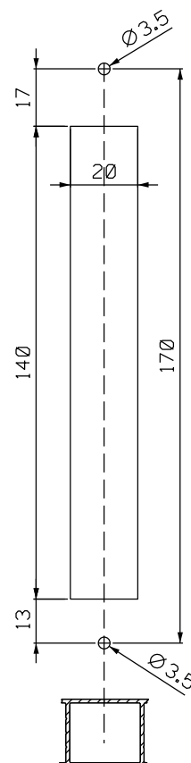
Usinagem - escala 1:2
