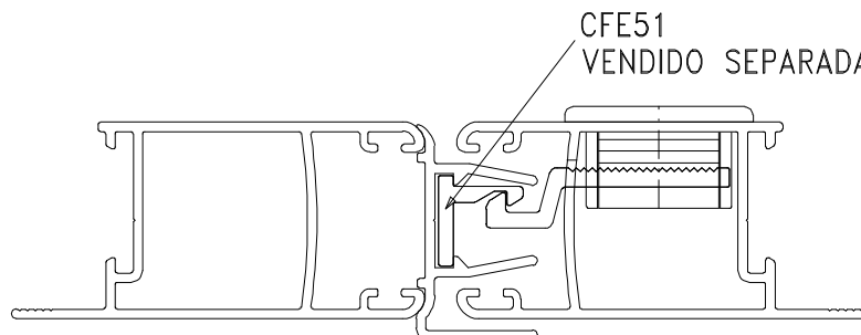
Instalação - escala 1:1
