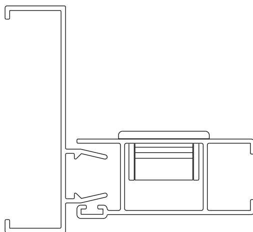
Instalação - escala 1:1
