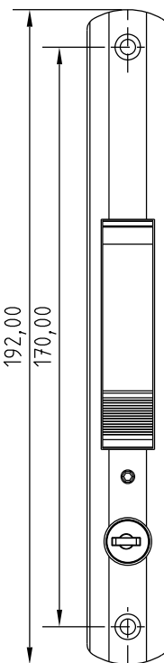
VISTAS - ESCALA 1:2
