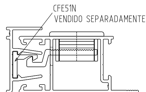
INSTALAÇÃO 1:1
