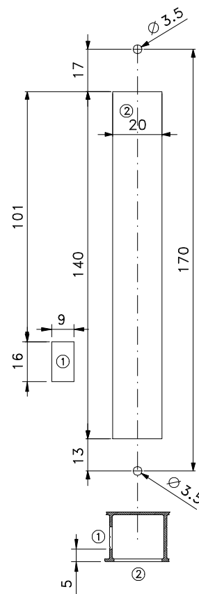
Usinagem – escala 1:2
