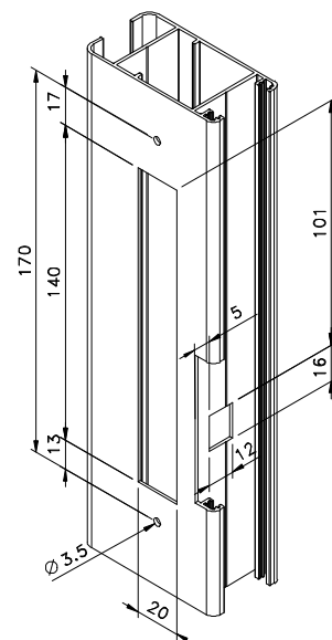
USINAGEM Sem escala
