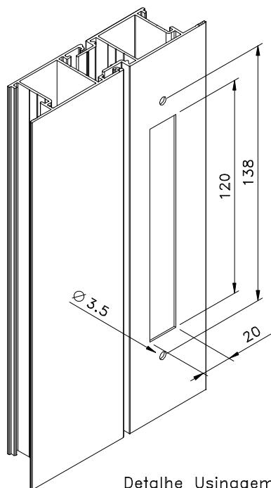
Detalhe Usinagem Sem escala
