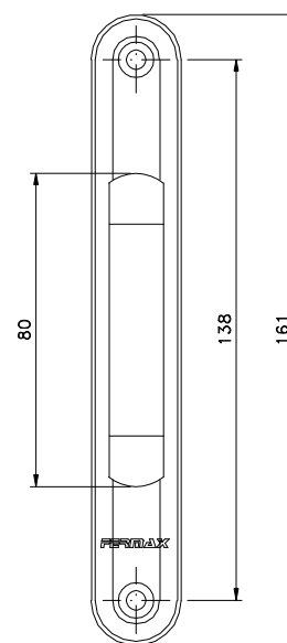
Vistas – escala 1:2
