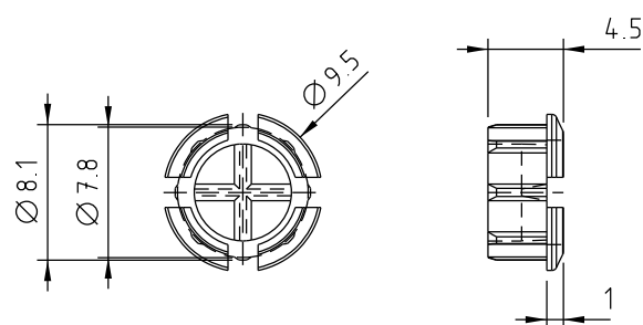
VISTAS ESCALA 2:1
