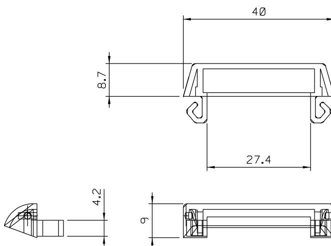
VISTAS ESCALA 1:1
