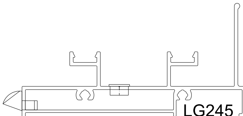
VISTAS ESCALA 1:1
