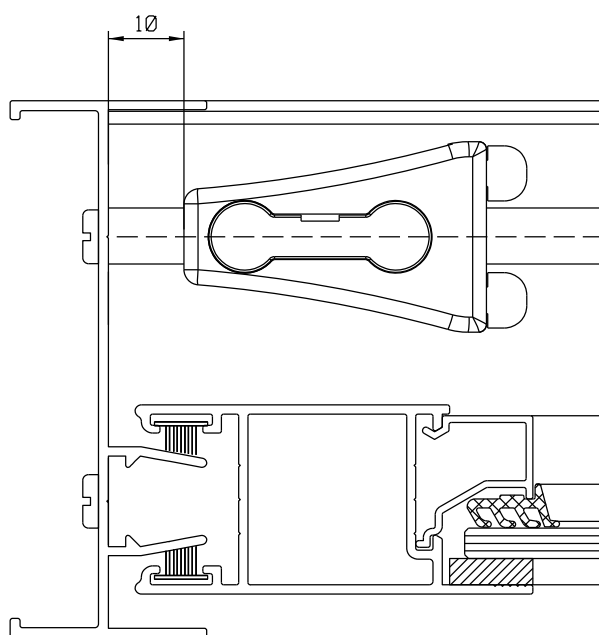
Instalação - escala 1:1
