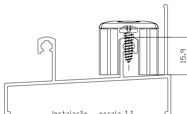
Instalação - escala 1:1
