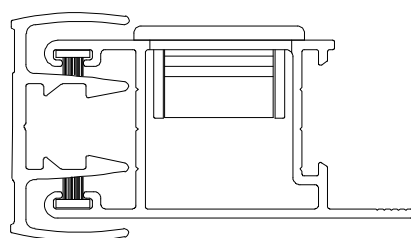
Instalação - escala 1:1
