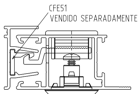
Instalação - escala 1:1
