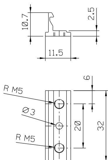
Vistas - escala 1:1
