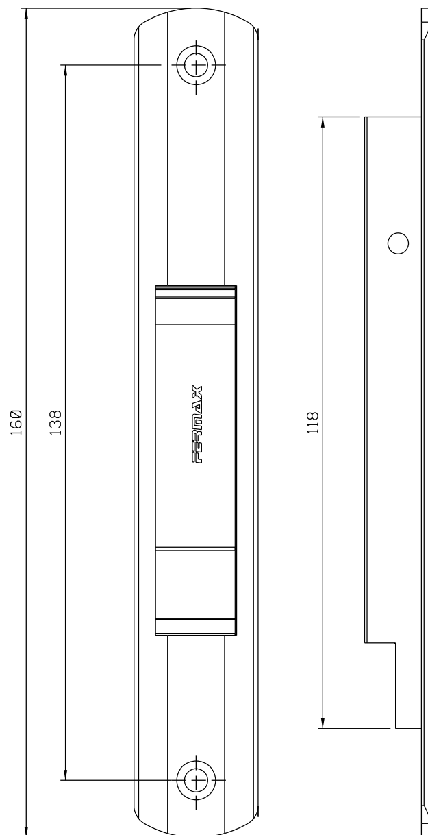
Vistas - escala 1:1
