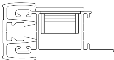
Instalação - escala 1:1
