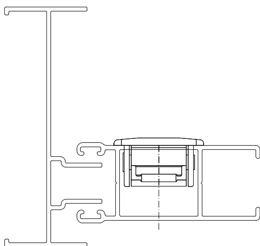
Instalação - escala 1:1
