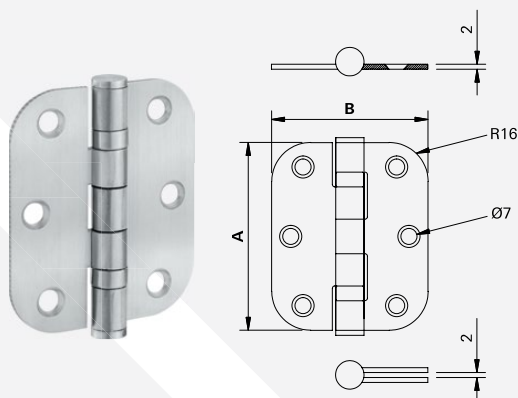
Dobradiça com Rolamento 3" x 2 1/2"
