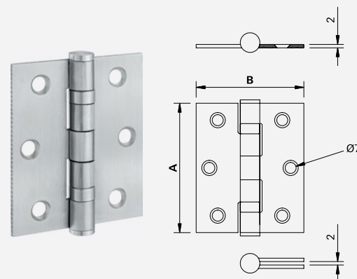
Dobradiça com Rolamento 3 1/2" x 3"
