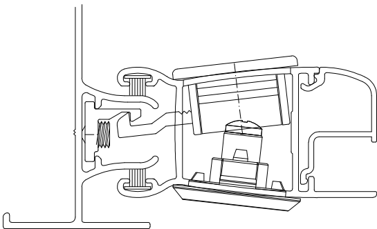
INSTALA**0 - ESCALA 1:1
