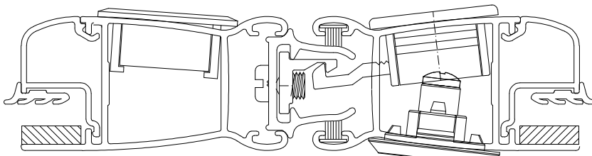
INSTALA**0 - ESCALA 1:1
