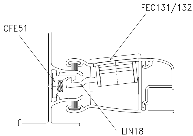
Instalação - escala 1:1
