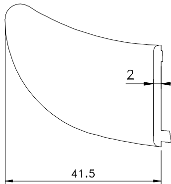
Vistas - escala 1:1
