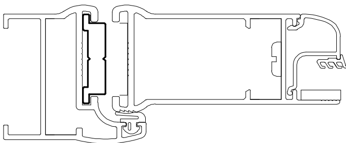
Instalação - escala 1:1
