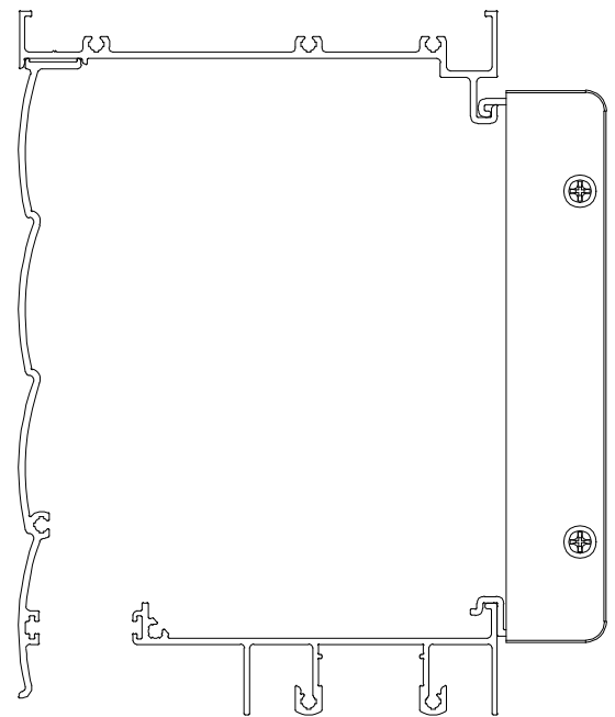
Instalação - escala 1:2
