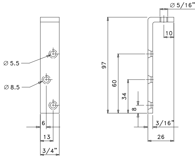
Vistas - escala 1:2
