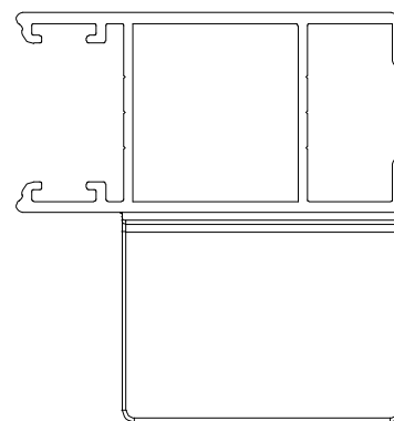
Instalação - escala 1:1
