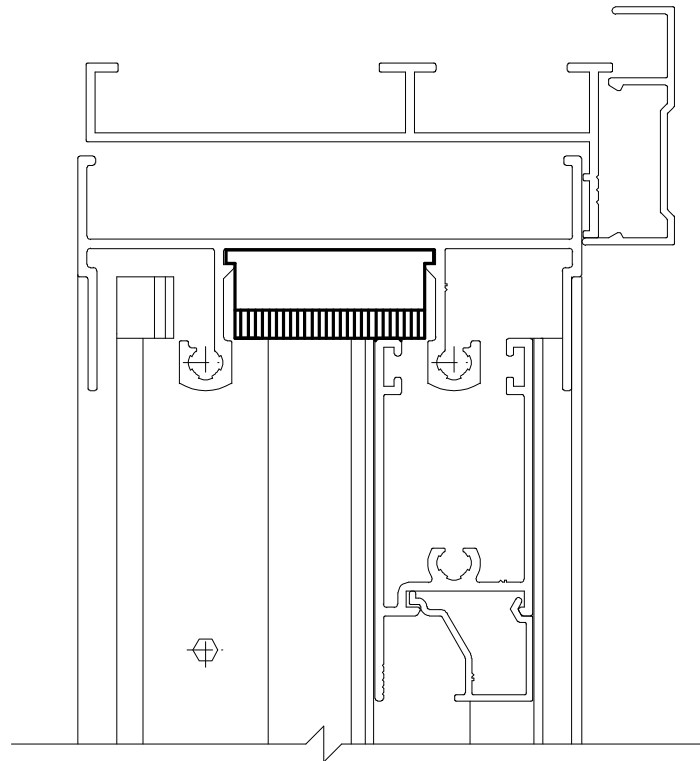
Instalação - escala 1:1
