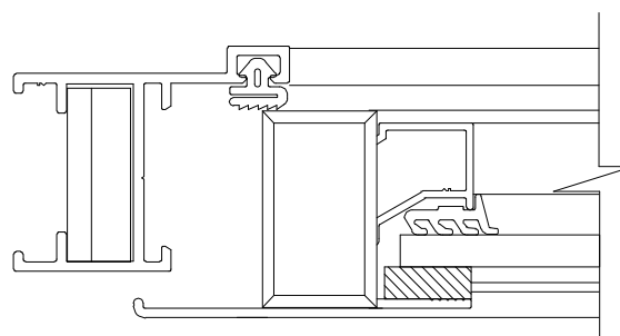
Instalação - escala 1:1
