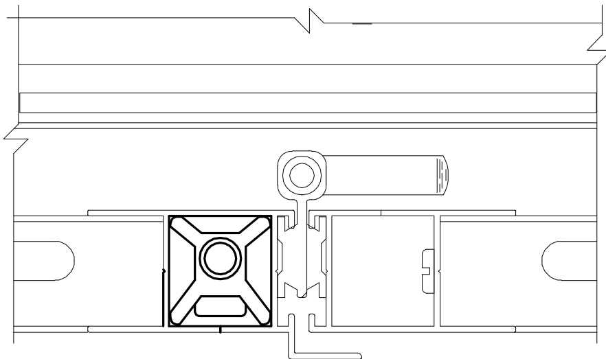
Instalação - escala 1:1
