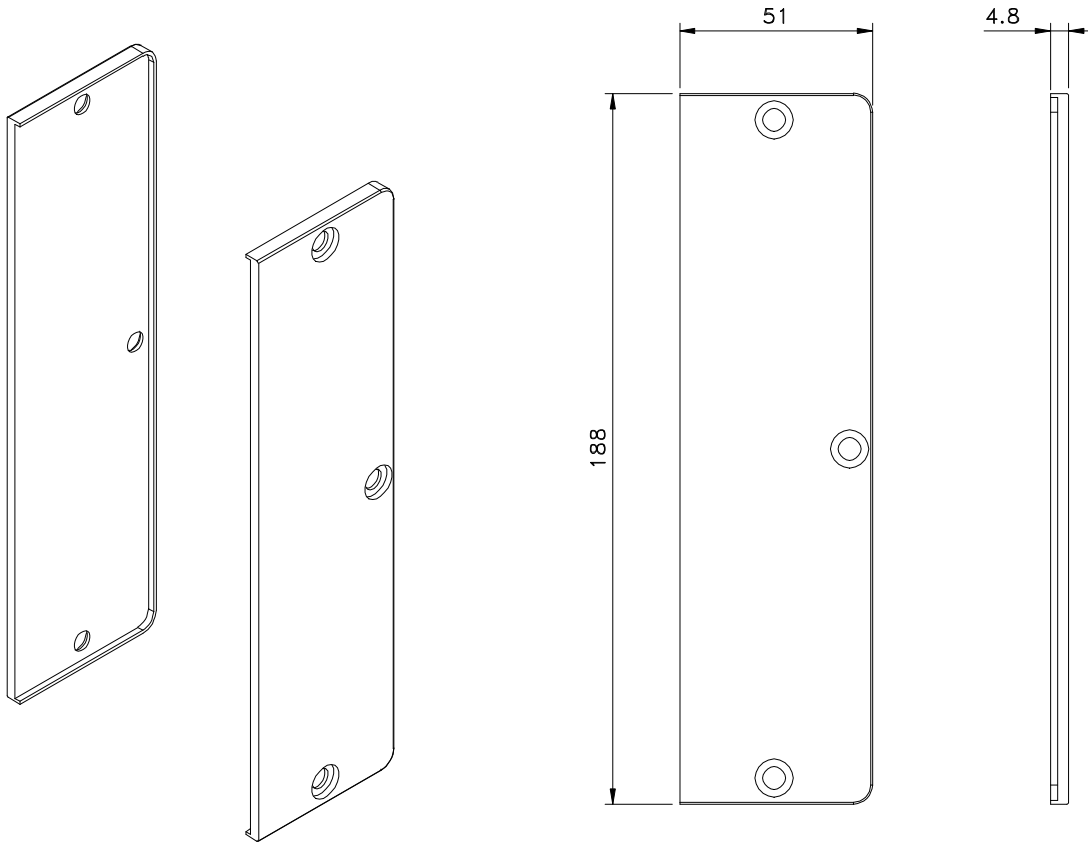
Vistas - escala 1:2
